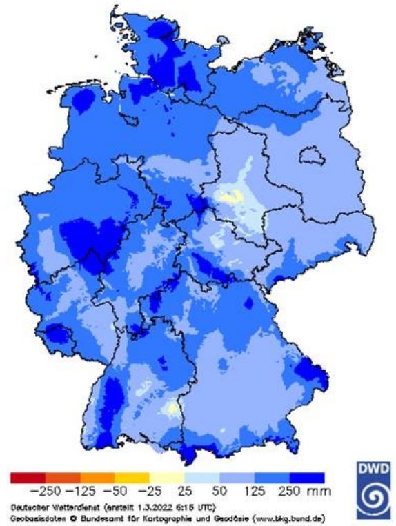
Klimatische Wasserbilanz 01.12.2021 – 28.02.2022
