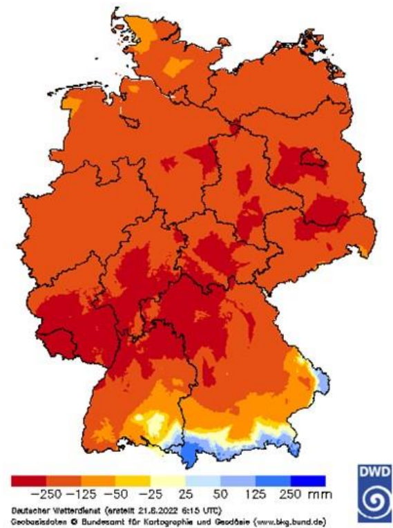
Klimatische Wasserbilanz 01.06.2022 – 20.08.2022
