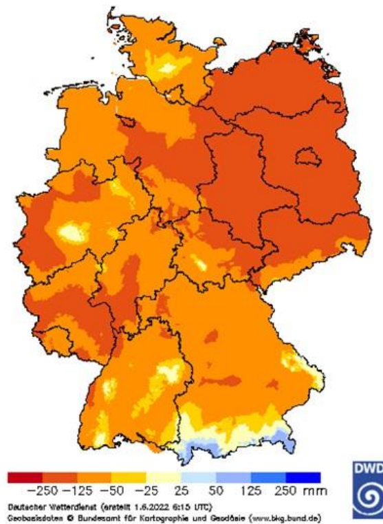
Klimatische Wasserbilanz 01.03.2022 – 31.05.2022
