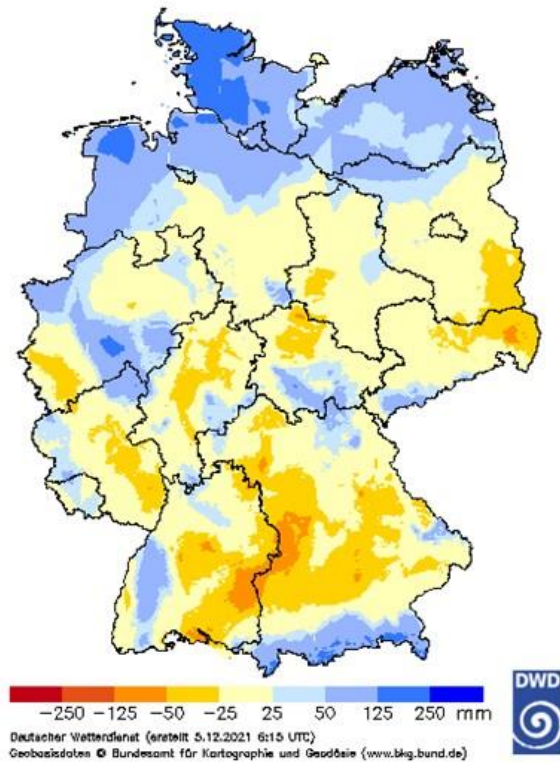
Klimatische Wasserbilanz 01.09.2021 – 30.11.2021
